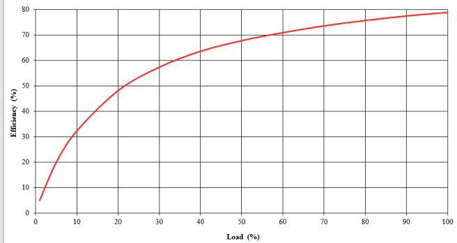
MGJ1D121503SC
