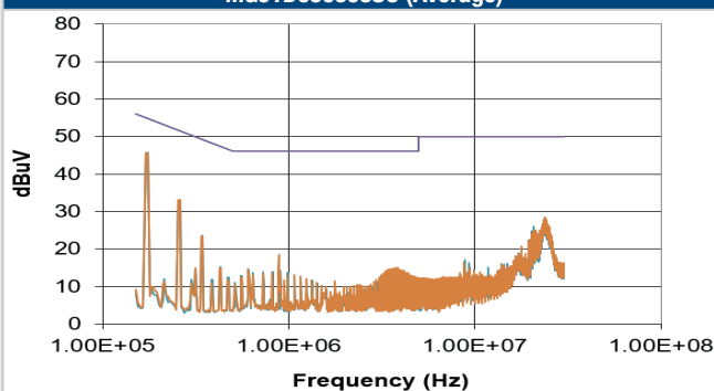
MGJ1D052005SC (Average)
