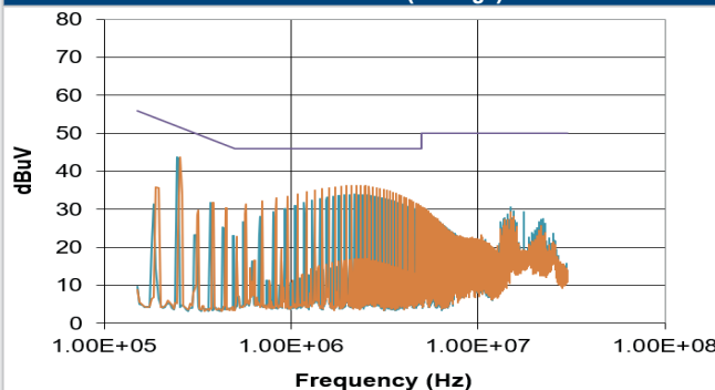
MGJ1D052005SC (Average)
